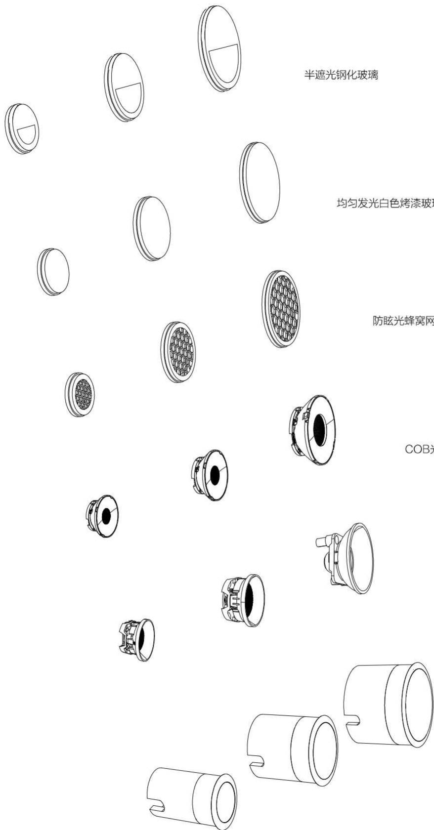
反光杯光学套件
